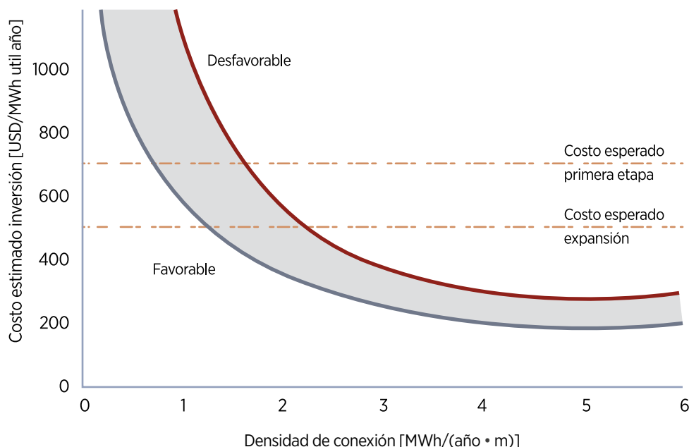
Figura 4-2: Costos de inversión específicos de la distribución del calor en función de la densidad de conexión, en un sistema de calefacción distrital. Fuente: Plnungshandbuch Fernwärme - Energie Schweiz (2017)
